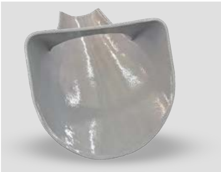
Coating met McCoat ST van trechter betonmixer voor verhogen slijtvastheid en verhogen flow van de natte beton
