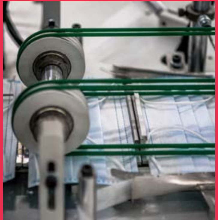
Rond- en V-snaren in PU
